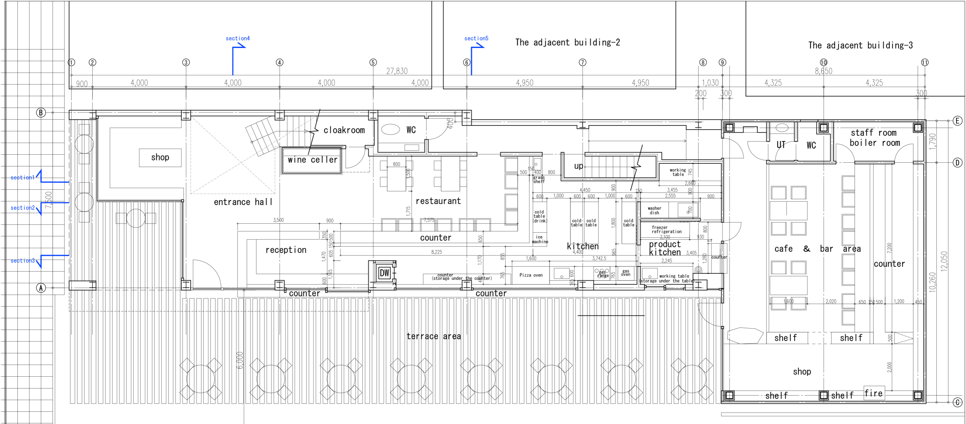
<1F plan>
